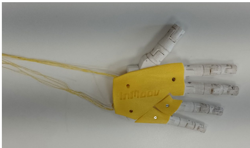
Figura 5 – Montagem da mão
