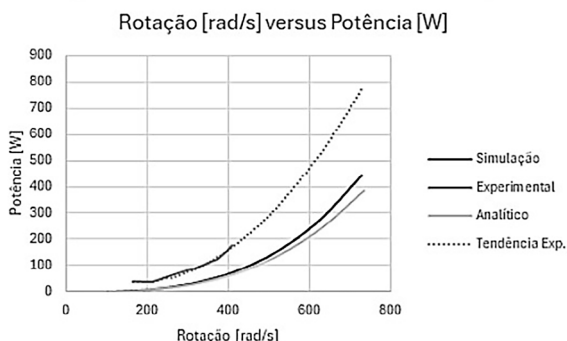
Figura 2 – Curvas de Potência versus Rotação
