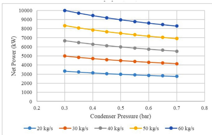
Figura 2 – Gráfico de potência líquida em função de pressão do condensador e vazão mássica de ciclopentano
