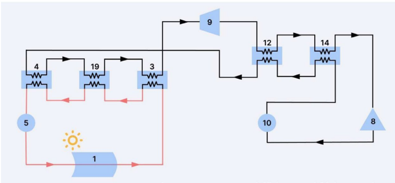
Figura 1 – Diagrama do ORC analisado
