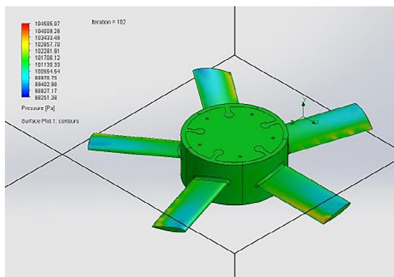
Figura 3 – Distribuição de pressão estática sobre as pás do rotor
