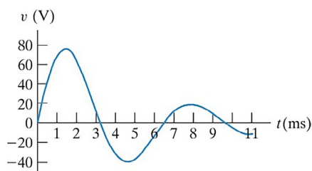
Figura 3 – Comportamento de um sinal em um circuito RLC
