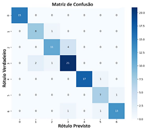
Figura 5 – Matriz de confusão do modelo unindo as medidas dos gases em porcentagem e as Razões de Rogers
