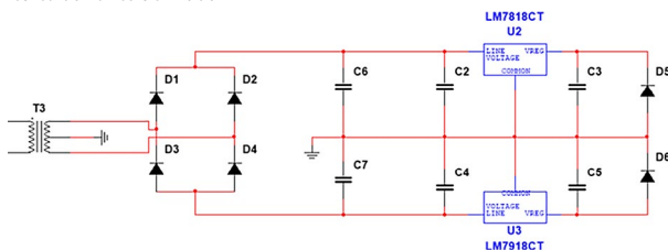
Figura 7 – Circuito da fonte utilizada
