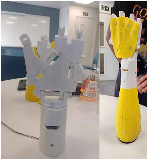
Figura 4 – Montagem do punho
