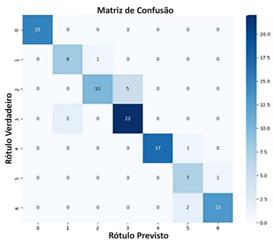
Figura 4 – Matriz de confusão do modelo usando a distribuição da base de dados balanceada
