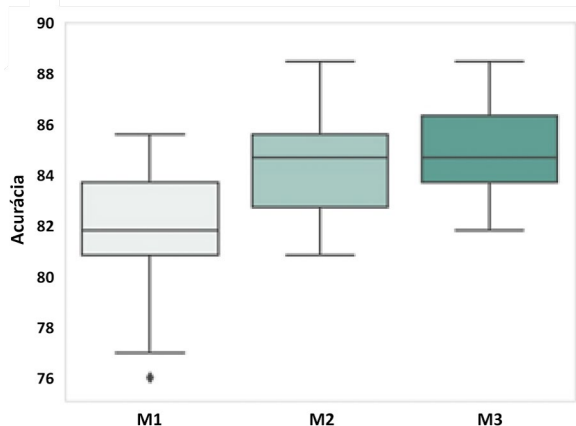
Figura 6 – Gráfico Boxplot da Acurácia dos Modelos
