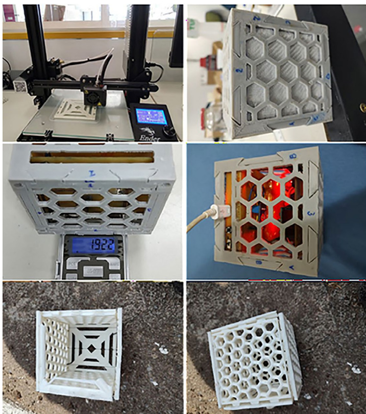
Figura 1 – Processo de fabricação, caracterização física e ensaio de impacto em queda livre a 10m
