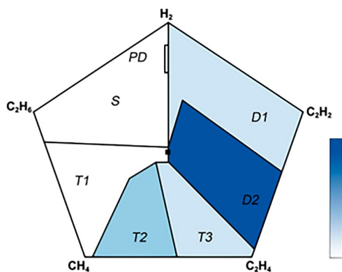
Figura 7 – Áreas do Pentágono de Duval com maior incidência de falhas adjacentes
