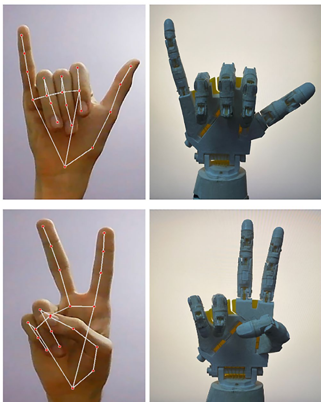
Figura 9 – Experimento 2– Movimentação simultânea de múltiplos dedos
