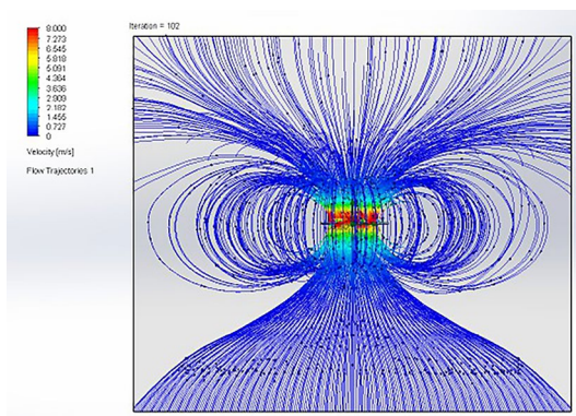
Figura 4 – Linhas de corrente representando a aceleração e o perfil de velocidade do escoamento
