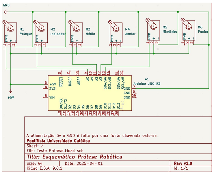
Figura 7 – Esquema do funcionamento dos motores
