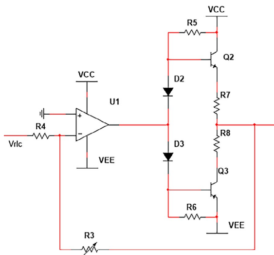
Figura 6 – Circuito de potência e controle de tensão
