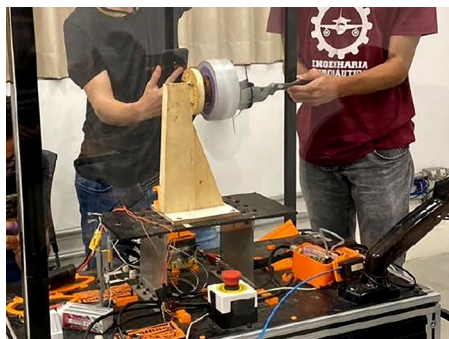
Figura 5 – Ensaios experimentais
