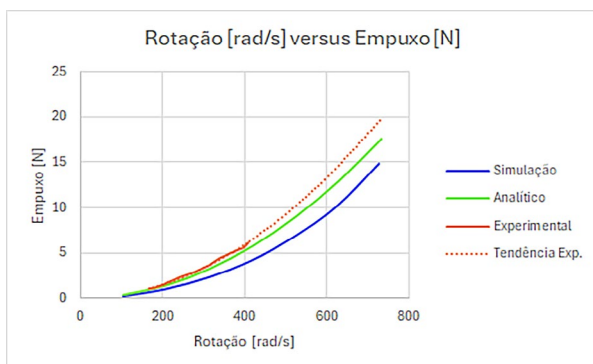
Figura 1 – Curvas de Empuxo versus Rotação
