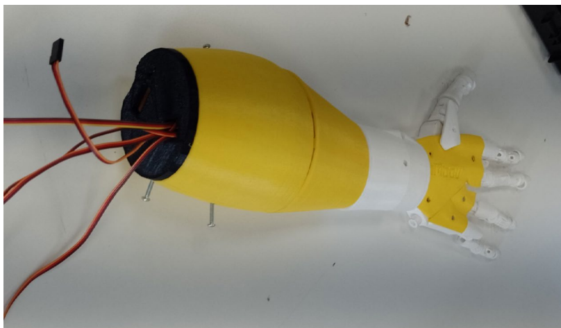
Figura 6 – Braço robótico
