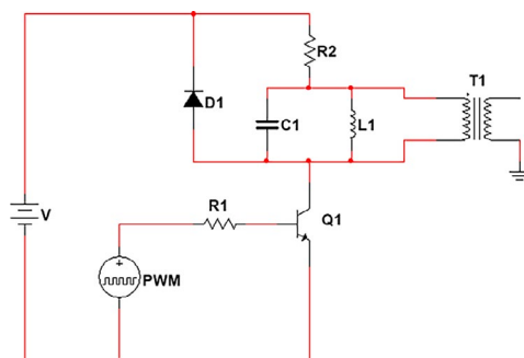
Figura 4 – Circuito RLC do protótipo
